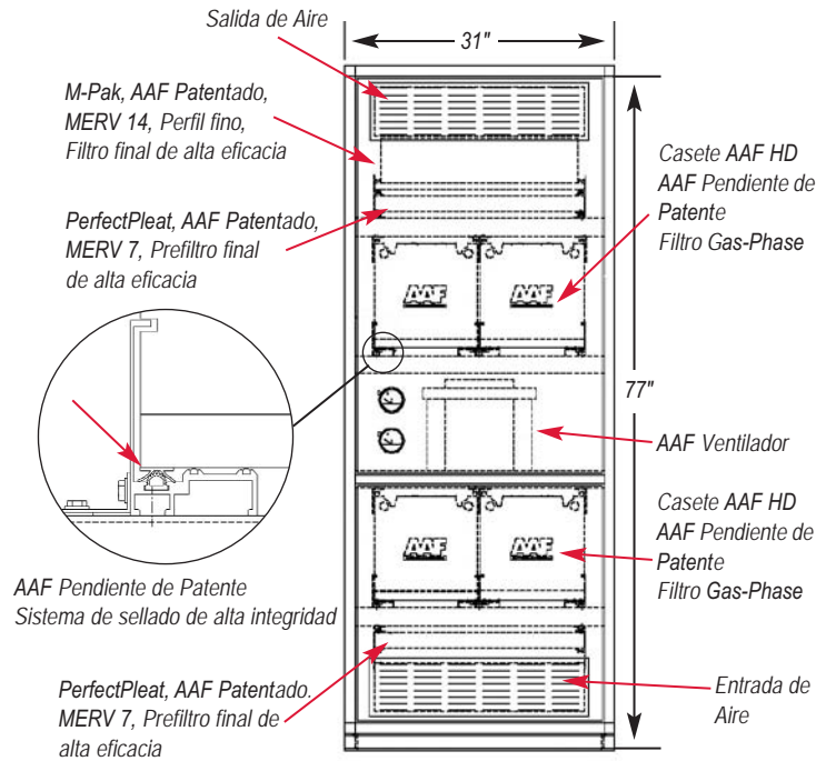
Esquema de sistema de Purificación vertical.
